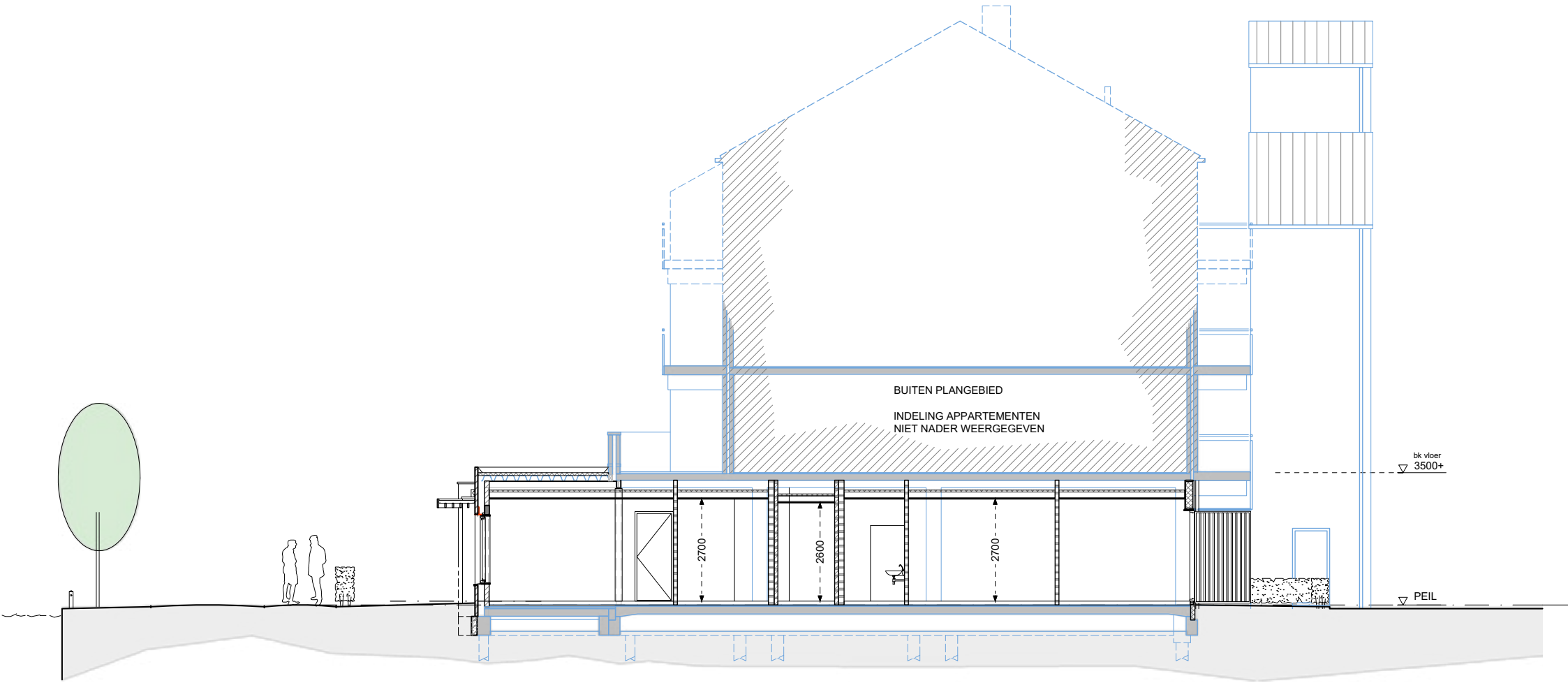
Doorsnede appartement en studio
