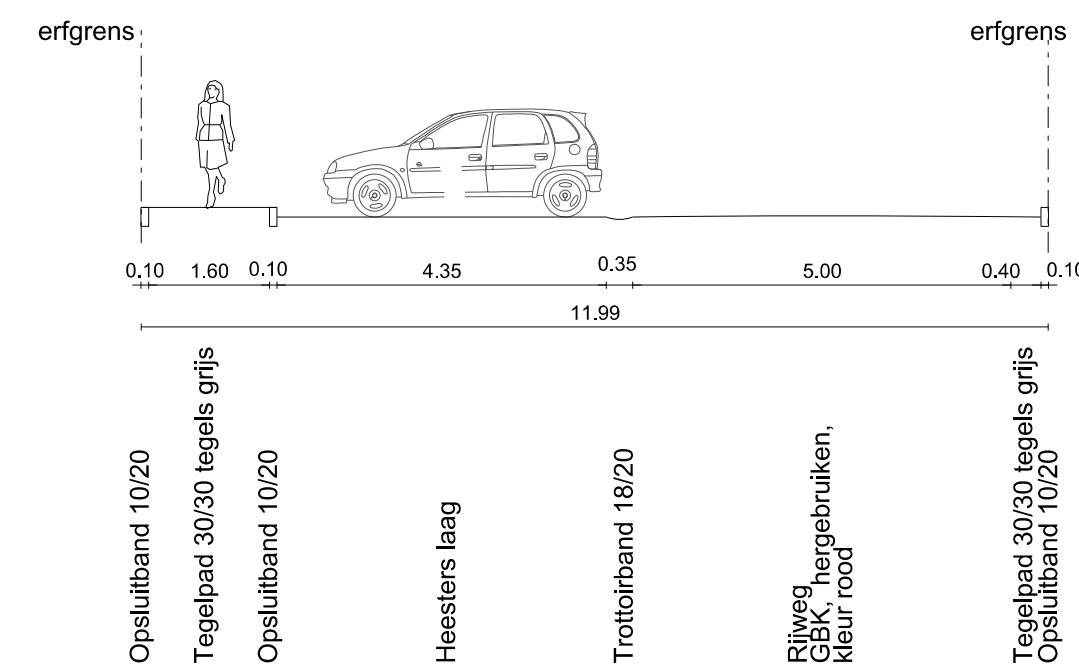
DWARSPROFIEL 12
