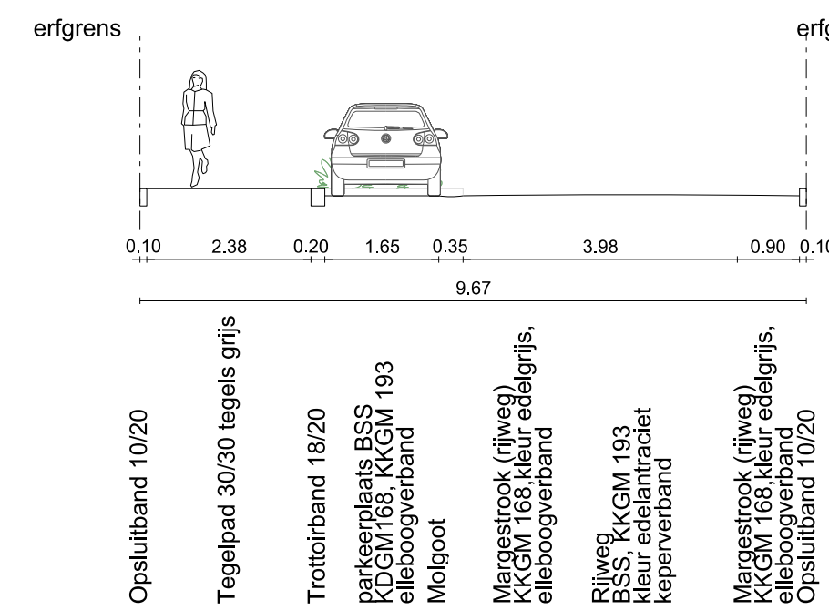
DWARSPROFIEL 3
