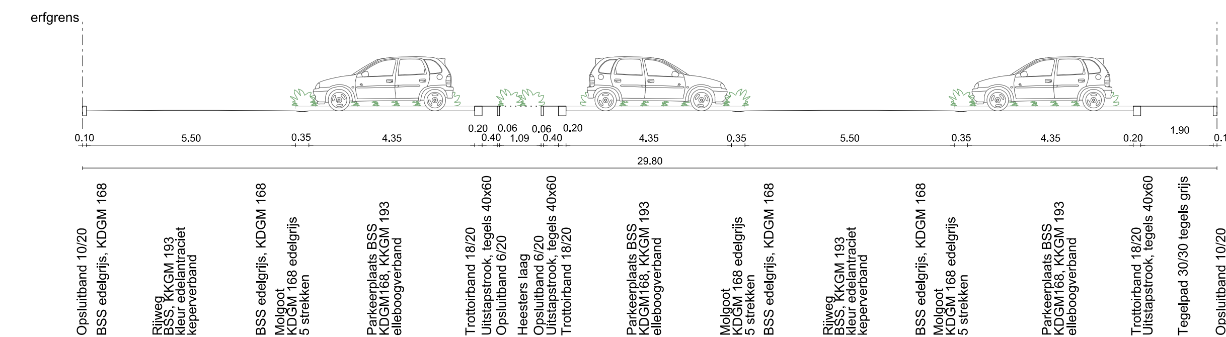
DWARSPROFIEL 8
