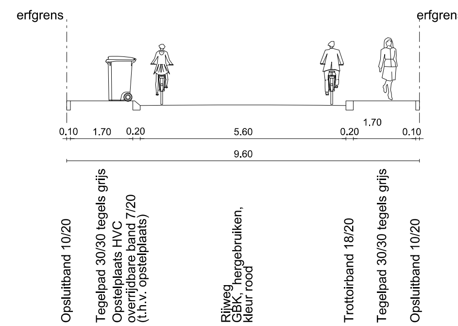
DWARSPROFIEL 5
