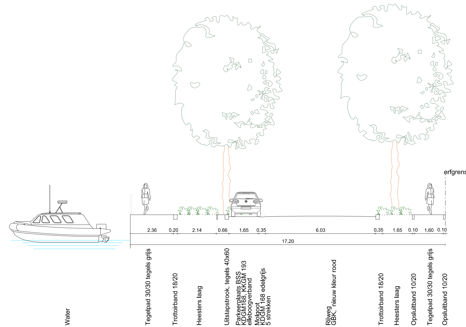
DWARSPROFIEL 6
