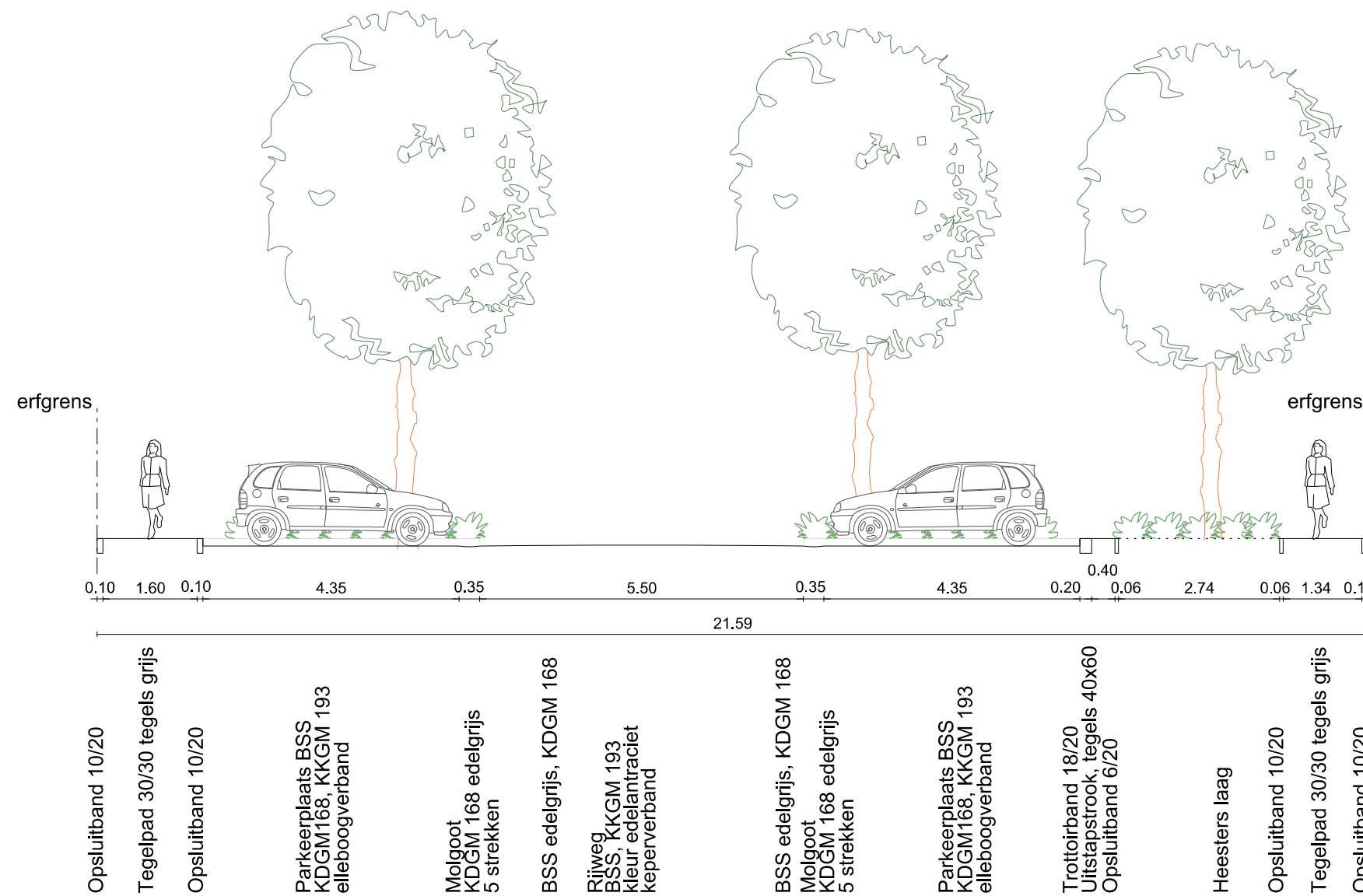
DWARSPROFIEL 11
