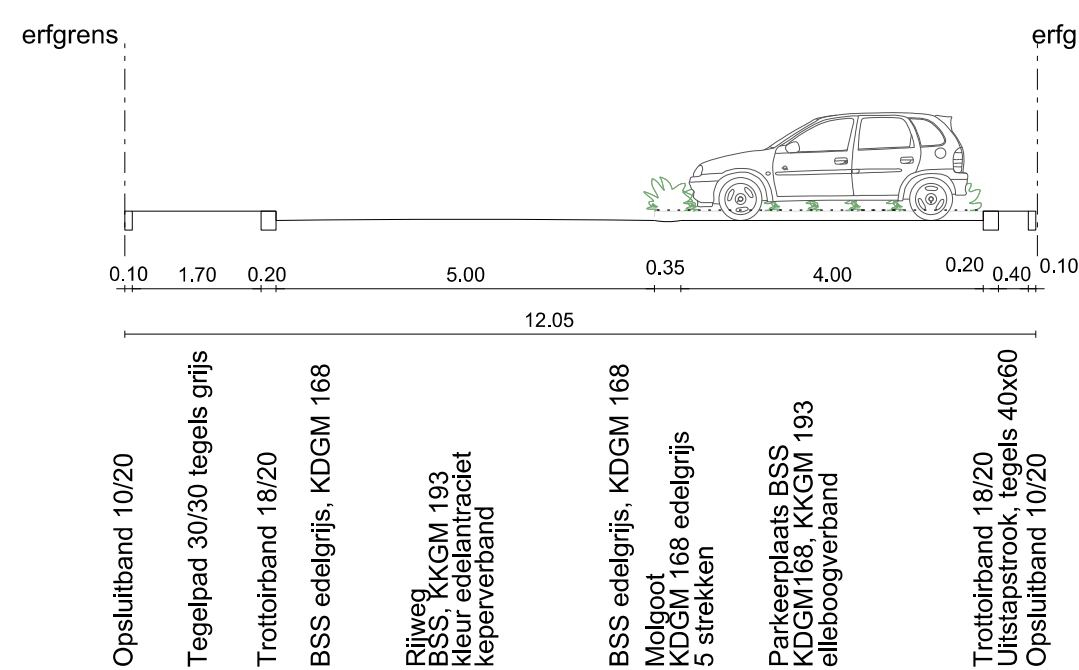
DWARSPROFIEL 7
