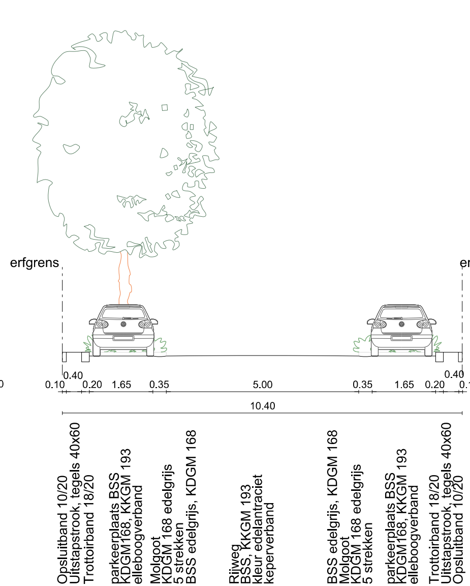
DWARSPROFIEL 13
