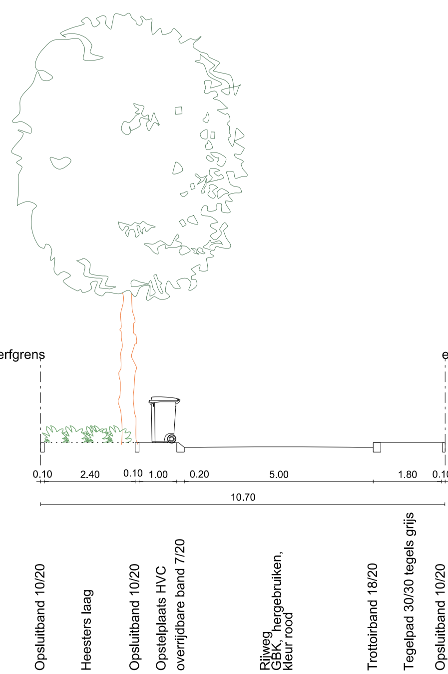
DWARSPROFIEL 1
