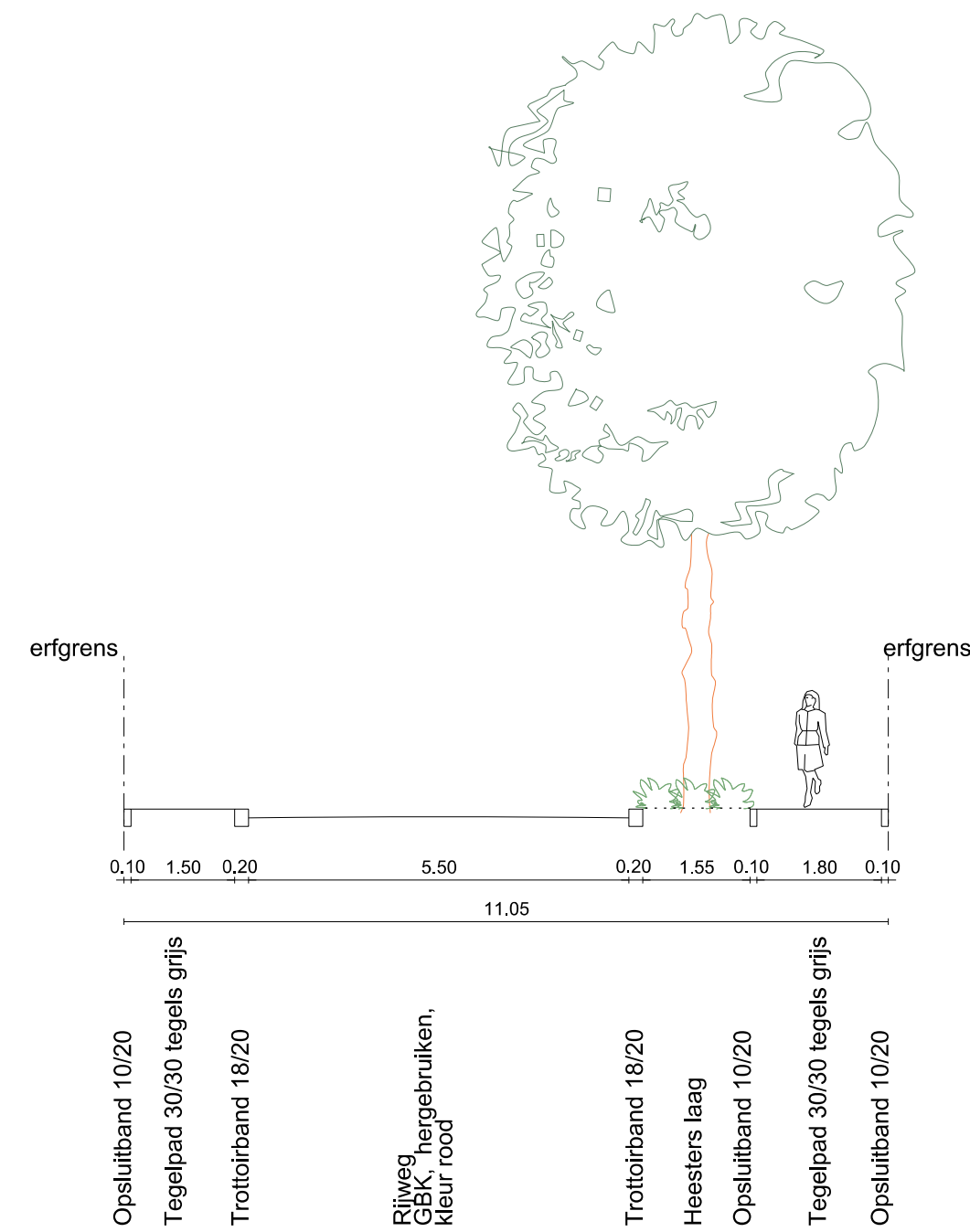
DWARSPROFIEL 2
