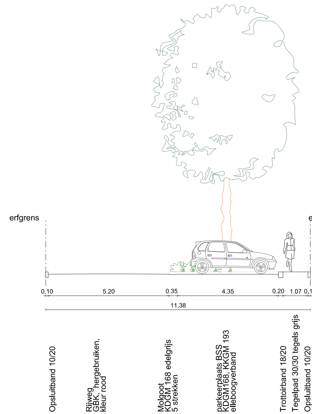
DWARSPROFIEL 4
