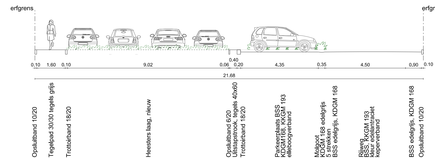
DWARSPROFIEL 10
