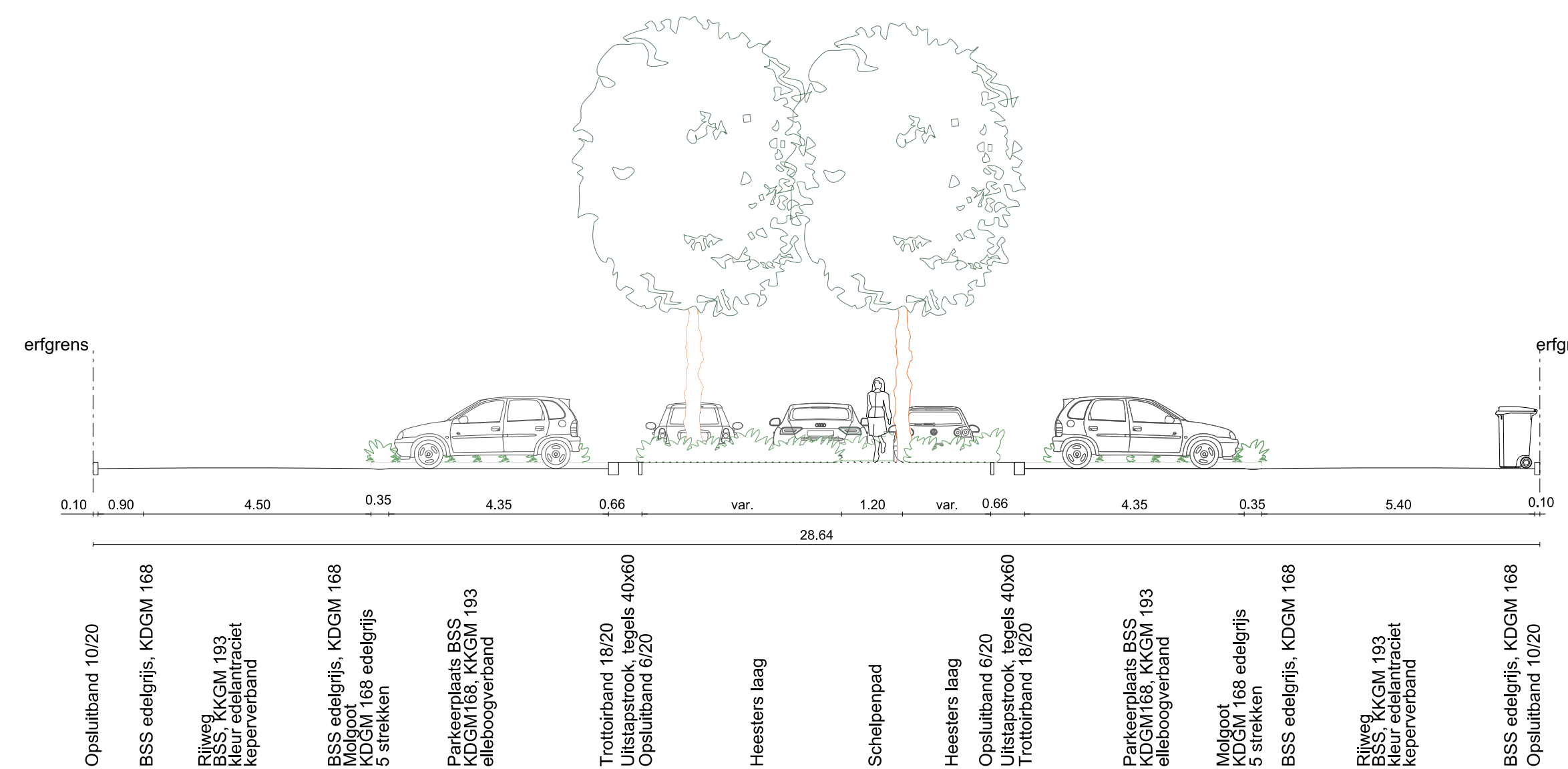
DWARSPROFIEL 14
