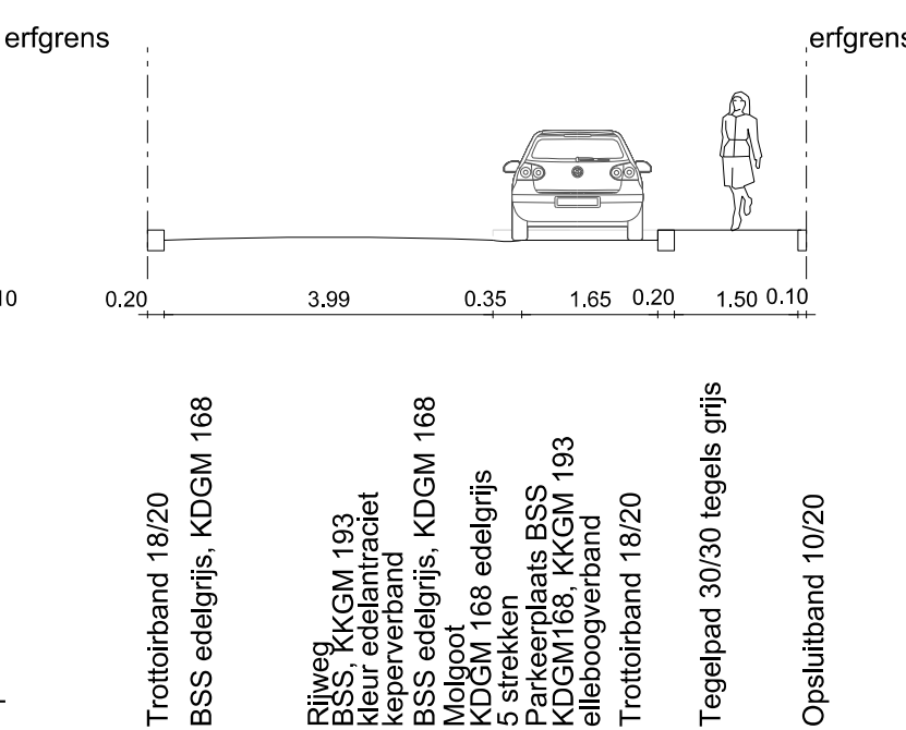
DWARSPROFIEL 9
