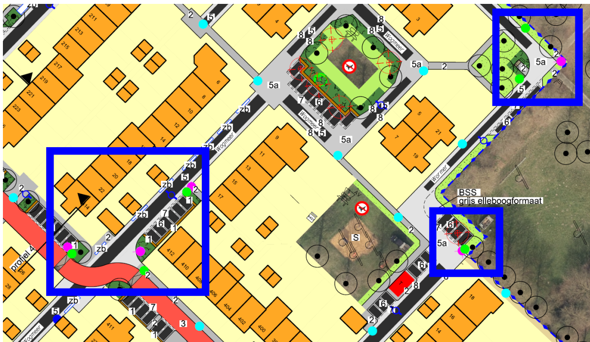
Afbeelding: uitsnede van de wijzigingen bij kruispunt Wogmeer met Ringdijk en Wormer.
